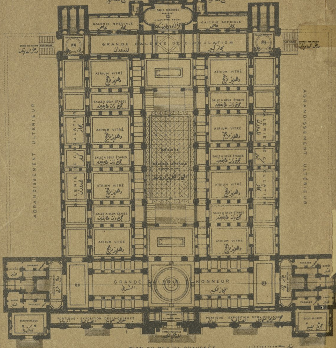
PLAN DU REZ-DE CHAUSÉE
