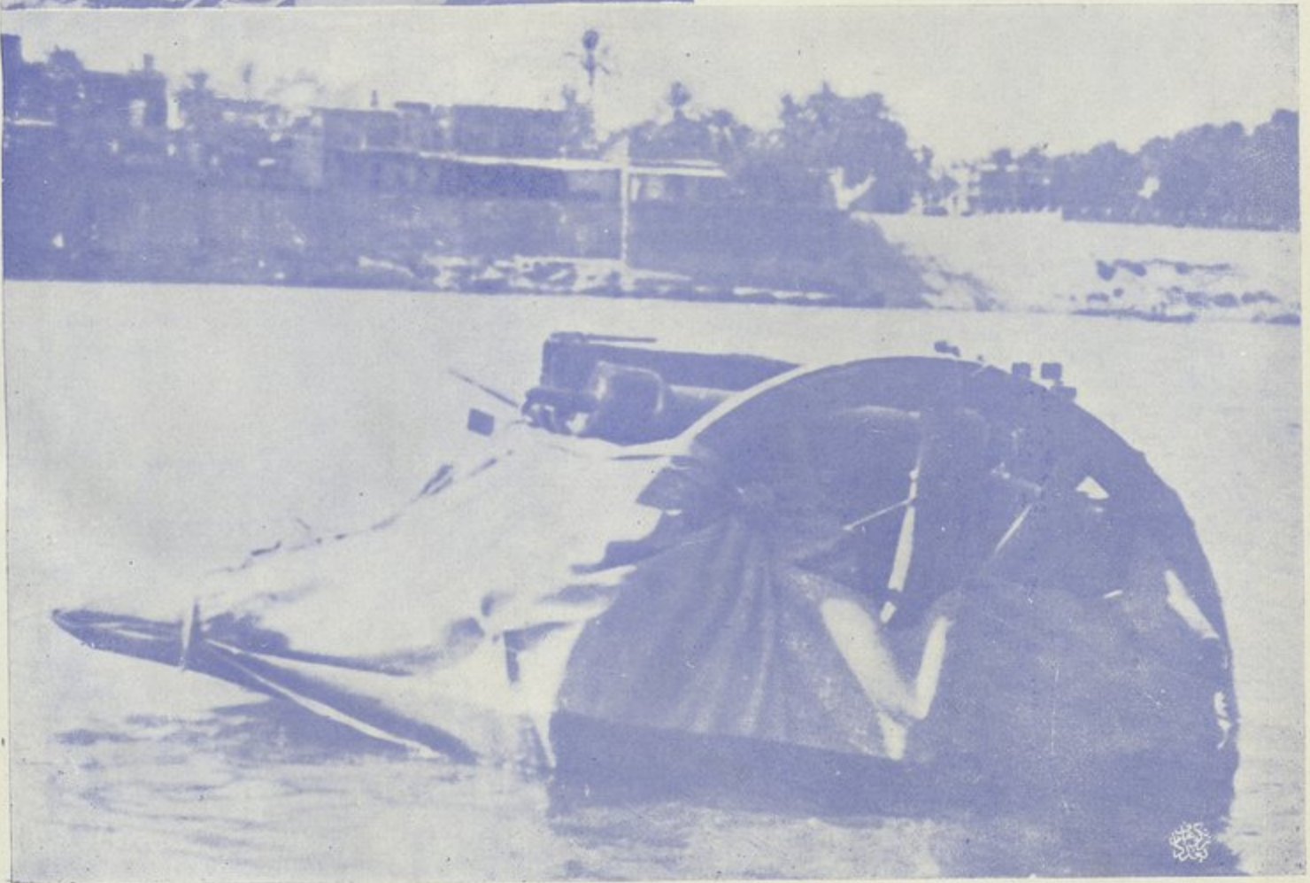
مدفع میونسرّاً علی قارب مطوی . A Gun crossing a River on a Folding Boat.
