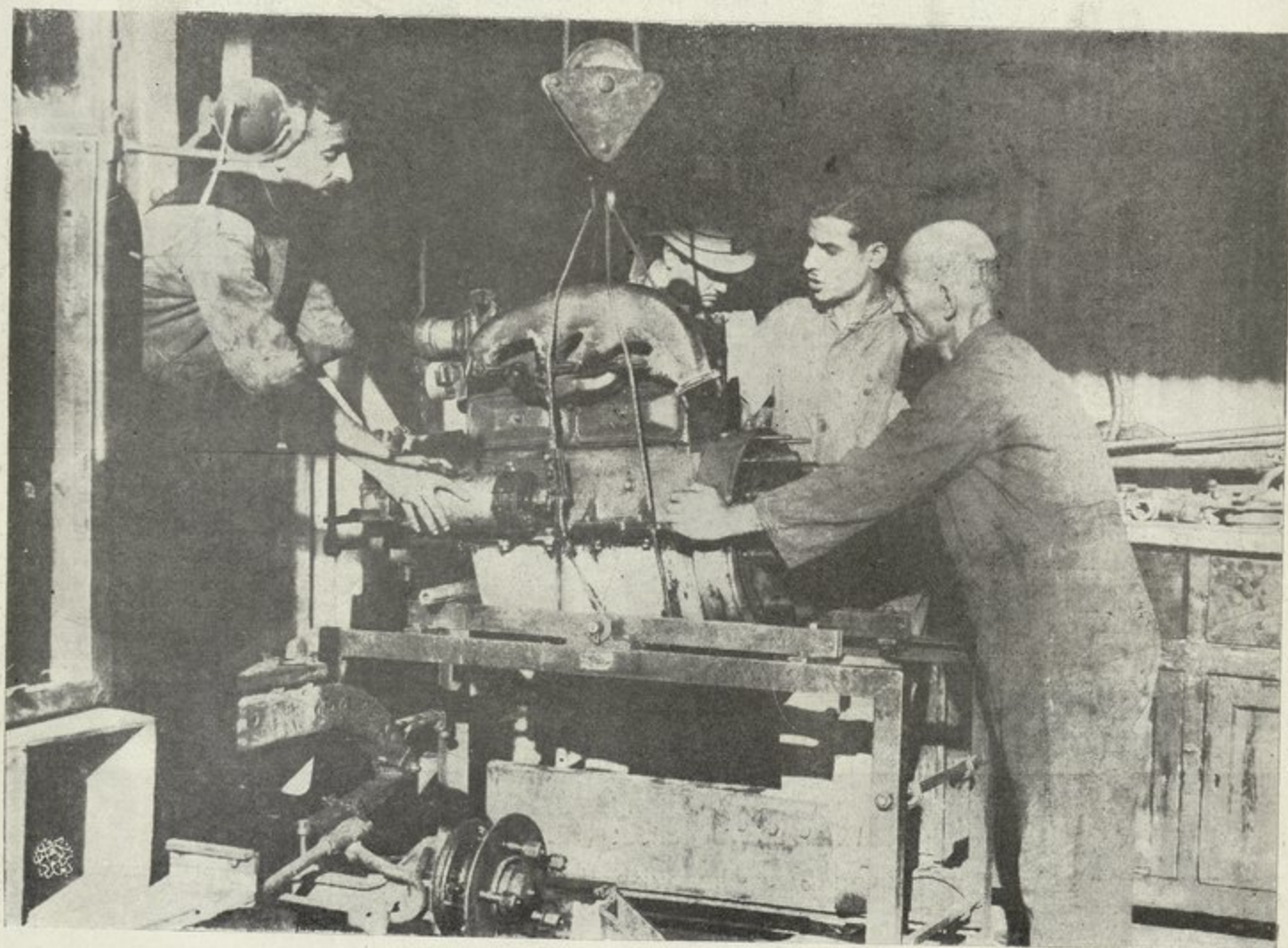
Chief Repair Workshop for the Army Mechanized Forces. معمل التصليح الرئيسي لآليات الجيش
