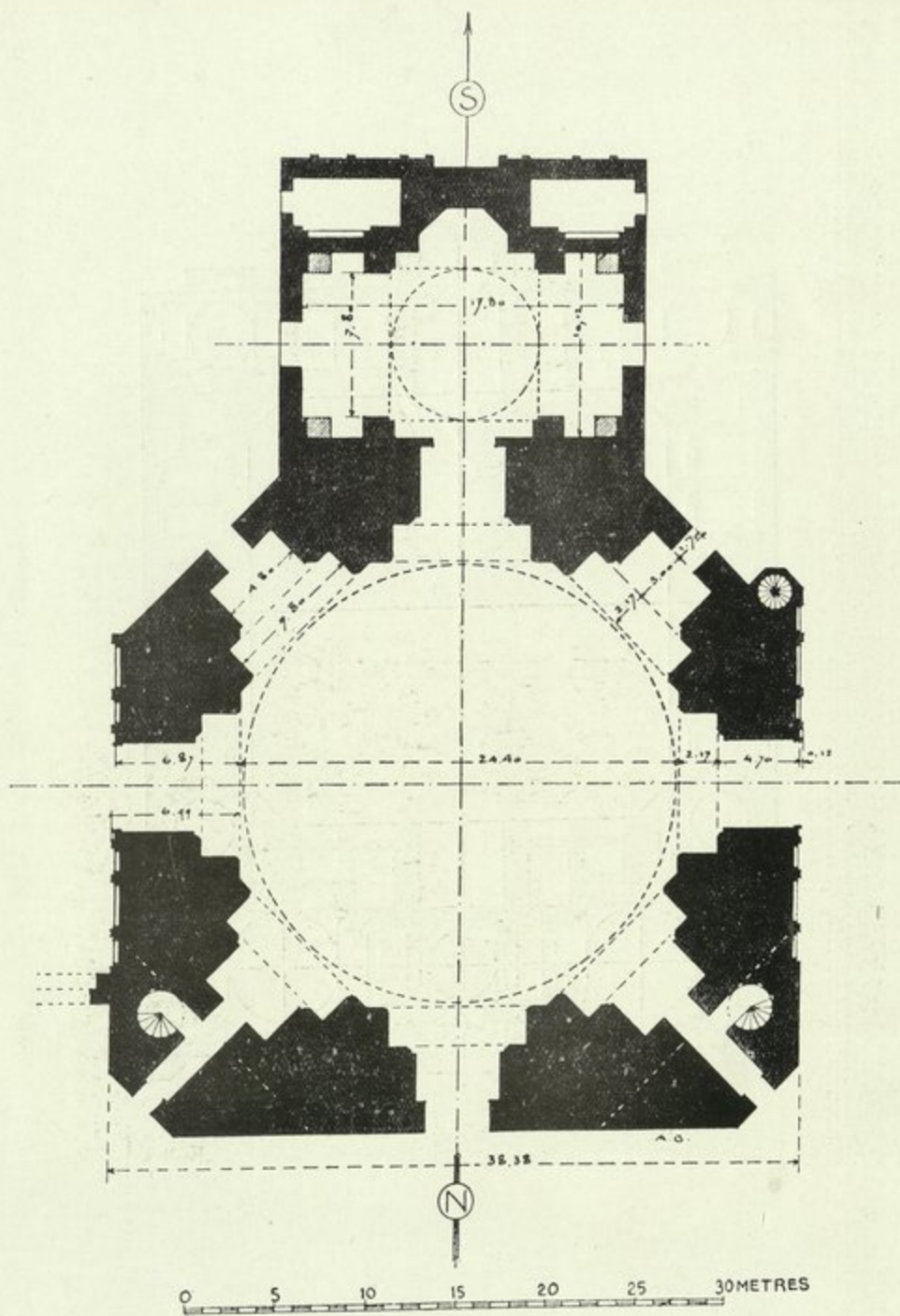
(شكل ٢٨) تخطيط ضريح الجانيوتوفى مدينة سلطانية (عن جودار)
