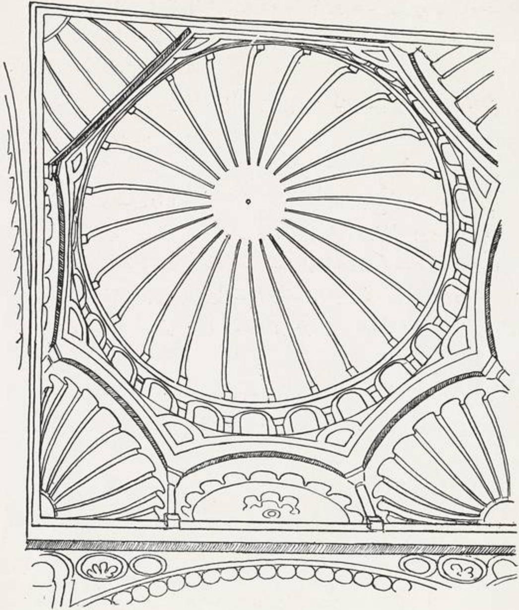
(شكل ٤٤) رسم تحليلي لهيكل قبة المحراب
