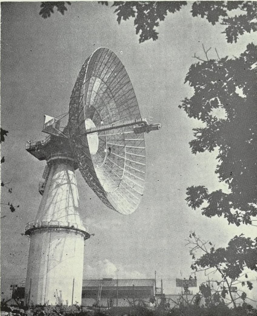
هوائي الرادار الضخم العائد للمؤسسة التكنولوجية في ماساشوست شمال بوسطن وقد ركب على برج طوله ٢٧ م ويبلغ قطره ٢٥,٥ مترا ويزن ٩٠ طنا وهو يكشف توابع البواحد القمرية .
