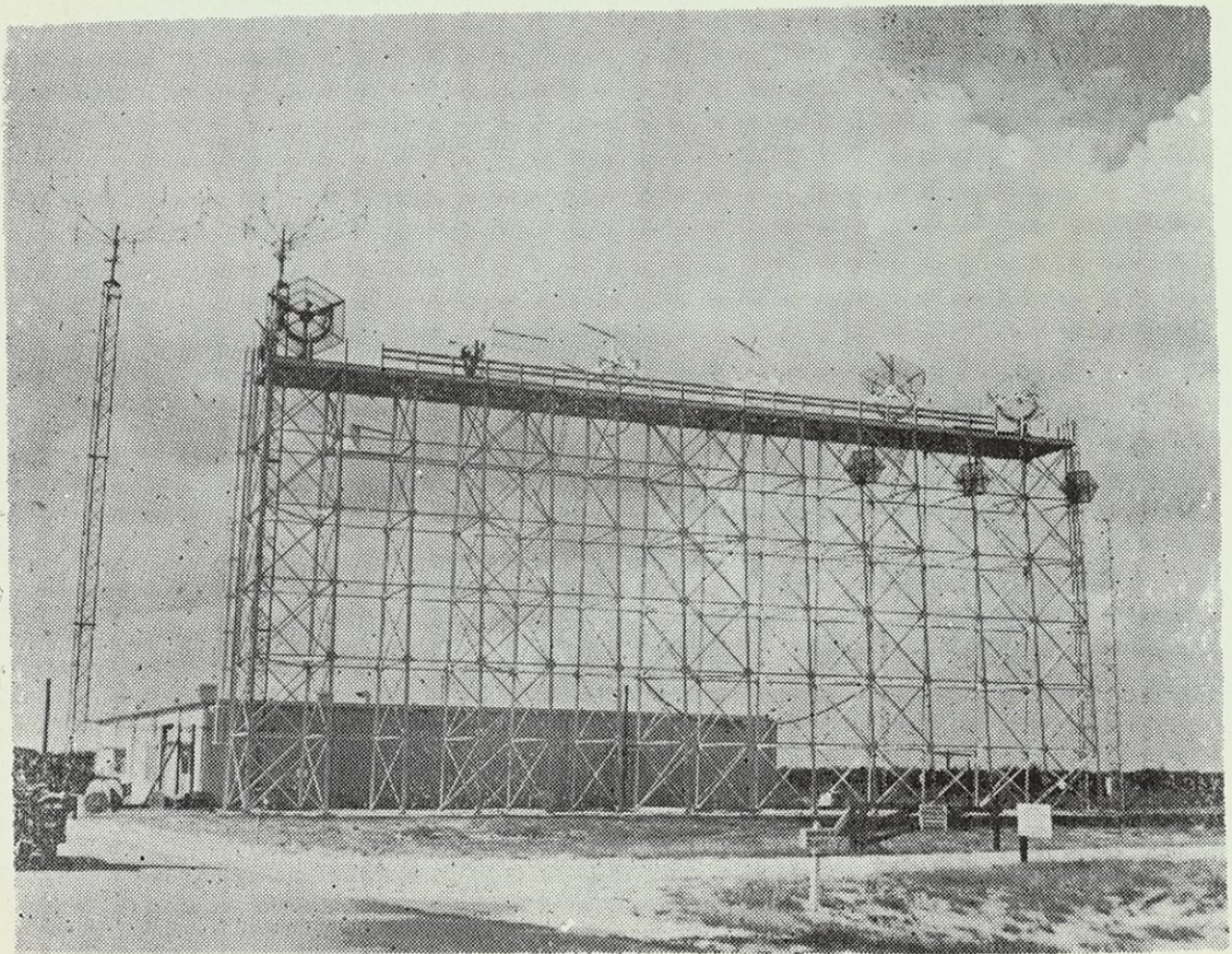
المحطة التلمترية في قاعدة رأس كانافيرال تسجل المعلومات الملتقطة من الرائد 1 ( 1958 ) .
