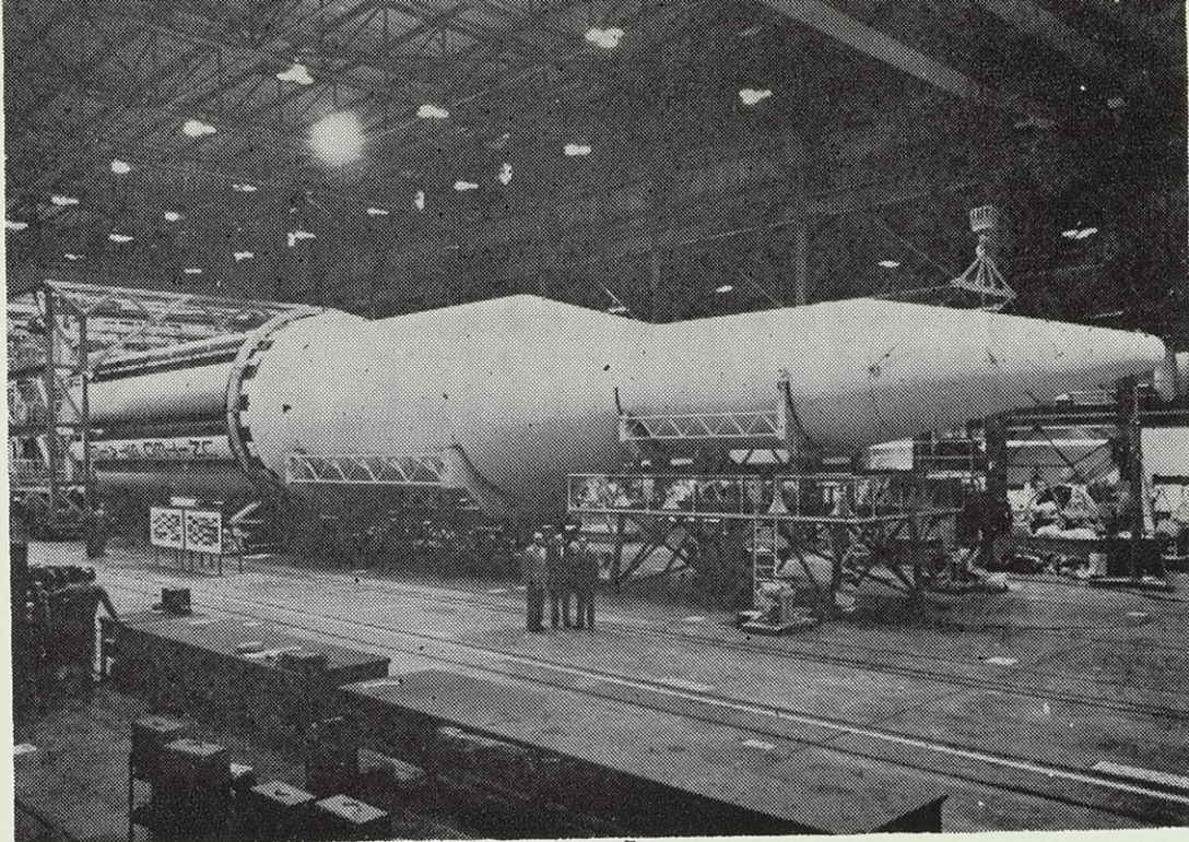
صاروخ زجل ( ٥٦ م ) في مرحلة الانتهاء تمهيدا لنقله الى مركز الاطلاق في رأس كانافيرال .
