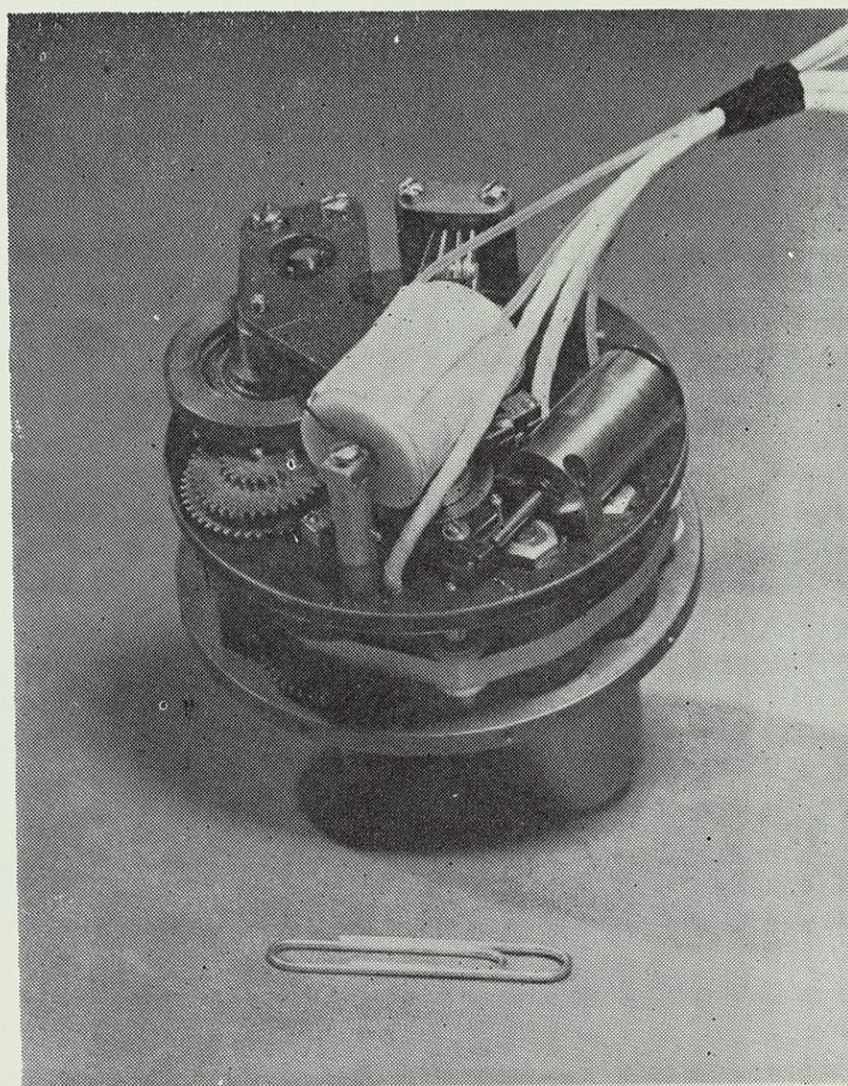
آلة التسجيل الصغيرة التي ركبت في تابع الكشاف ٣ ويبلغ عرضها ٦,٥ سم ووزنها ٢٢٥ غرام . وقد وضع امام الجهاز ( شكلة ورق ) لتقدير حجم الجهاز بالمقارنة .
