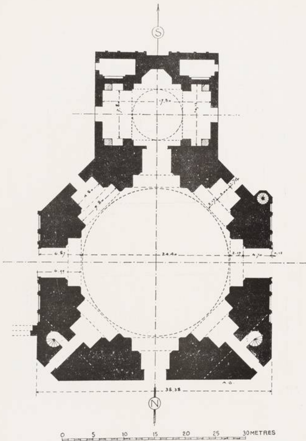
(شكل ٢٨) تخطيط ضريح الجاينوفى مدينة سلطانية (عن جودار)
