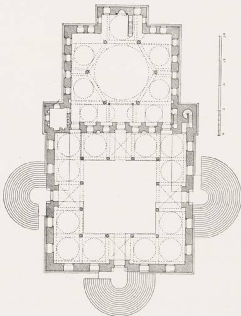
مسقط أفق
