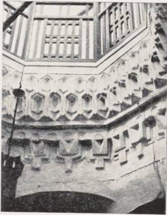
مقرنصات المنسور
