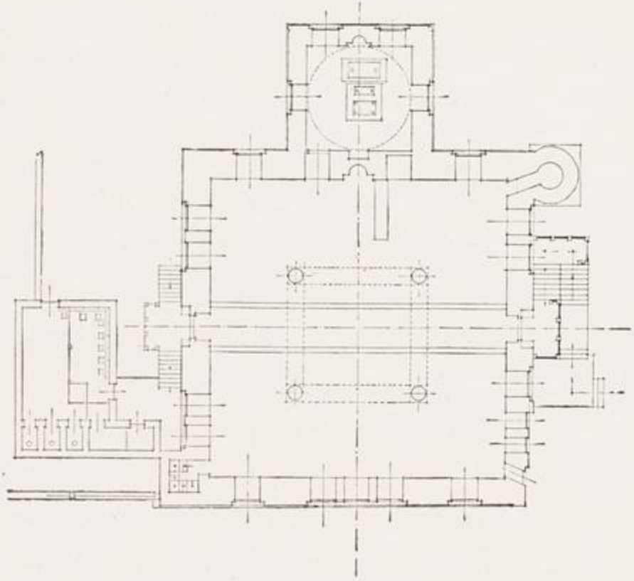
مسقط أفق
