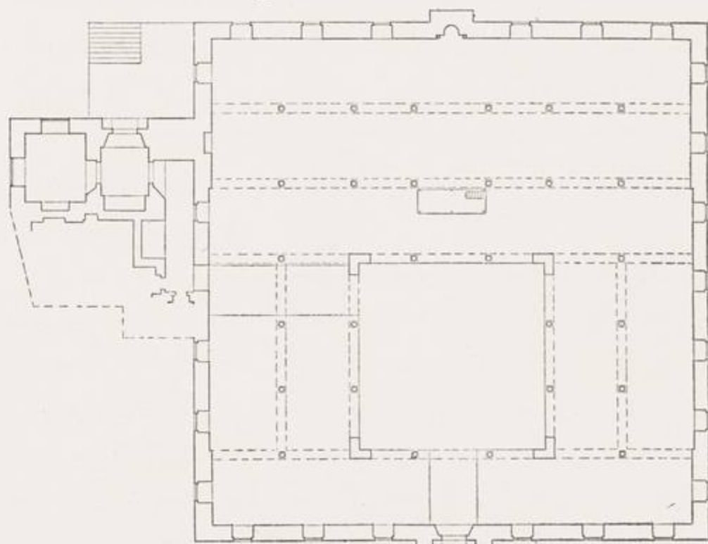
مسقط أفق
