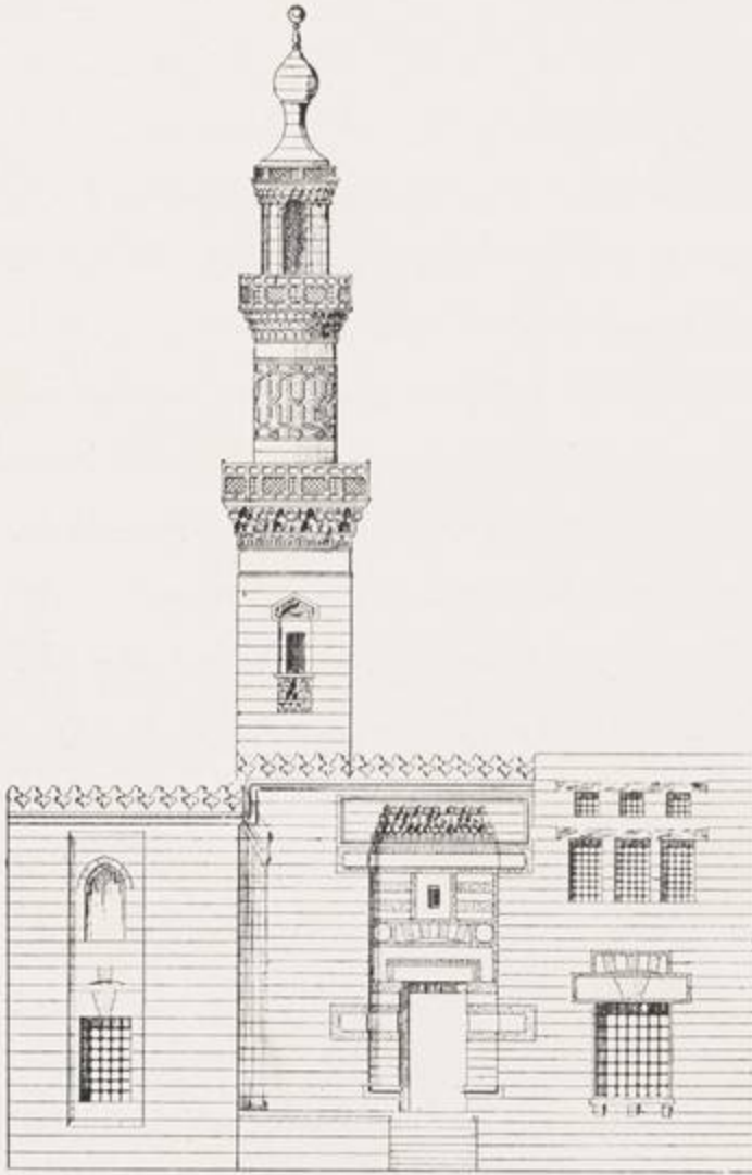
المدخل والمنارة
