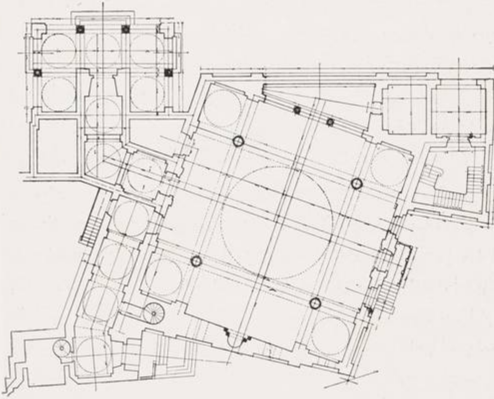
مسقط افق
