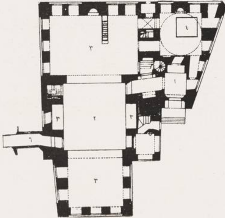
مقطع أفق
