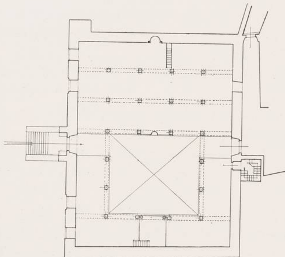
مسقط أفق
