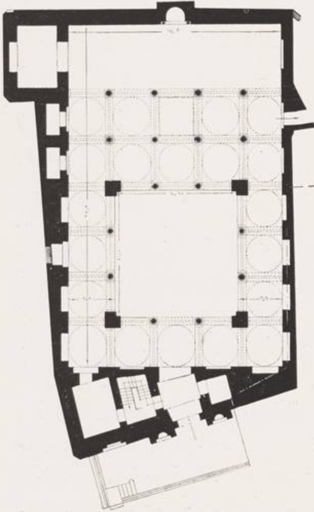
مسقط أفق
