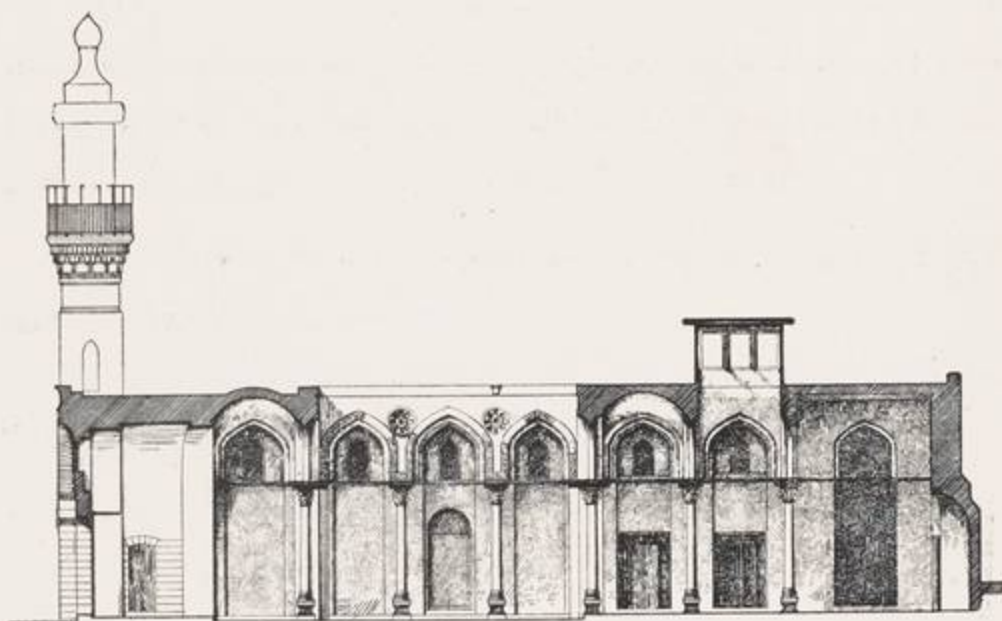
قطاع رأسي
