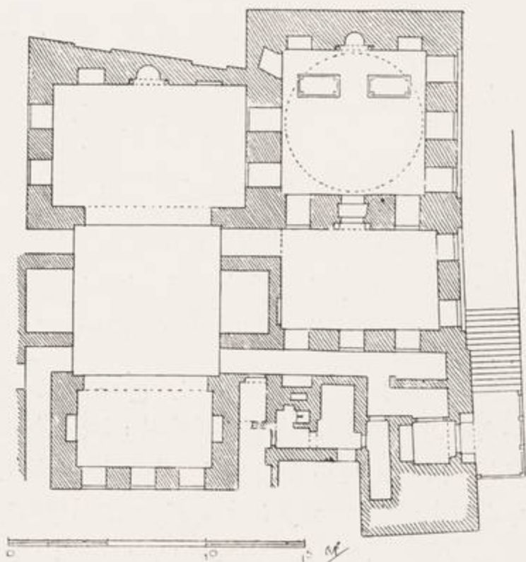
مسقط أفق
