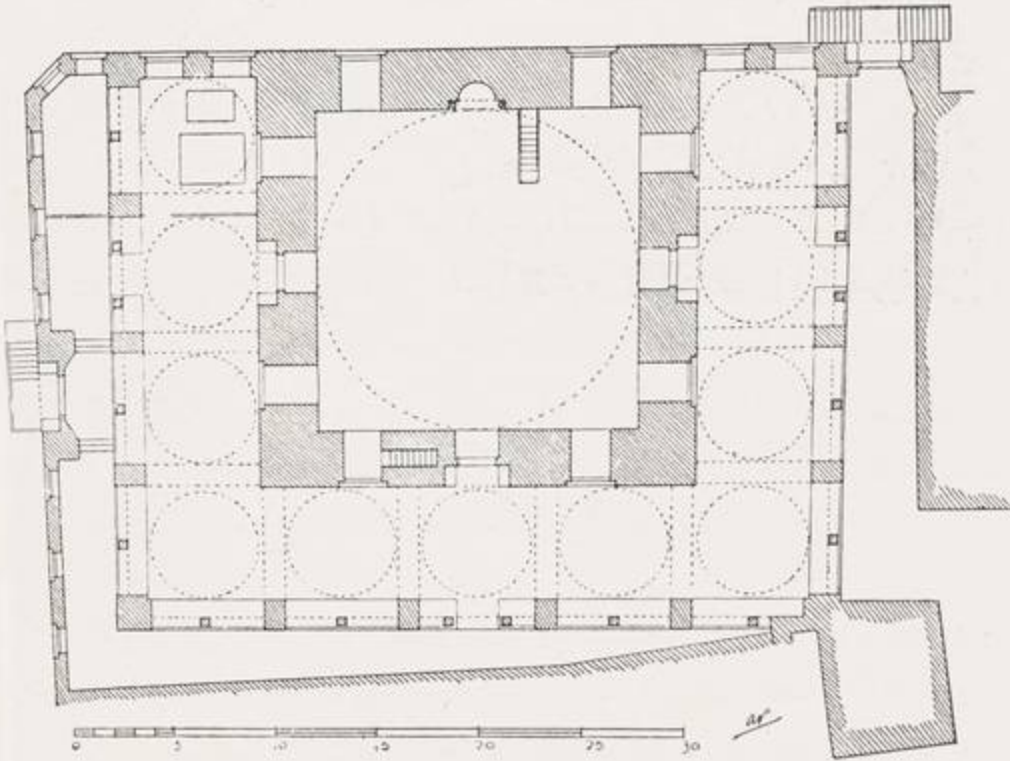
مسقط أفق
