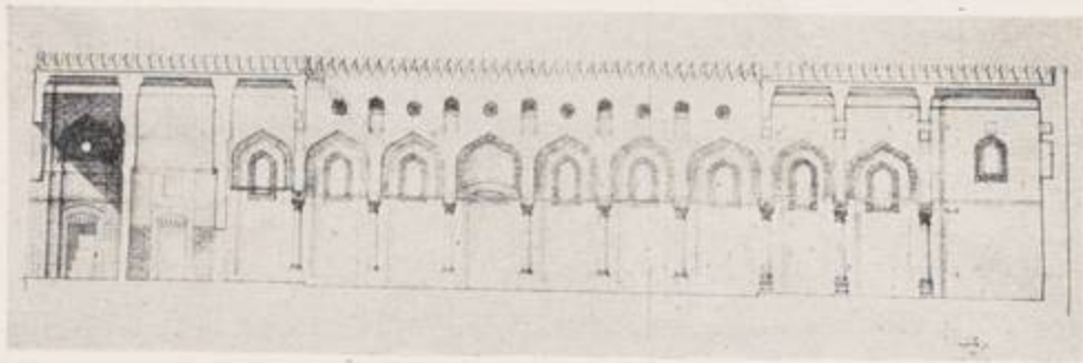
قطاع طولى
