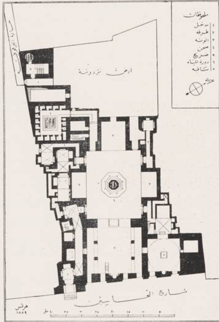
مسقط أفق
