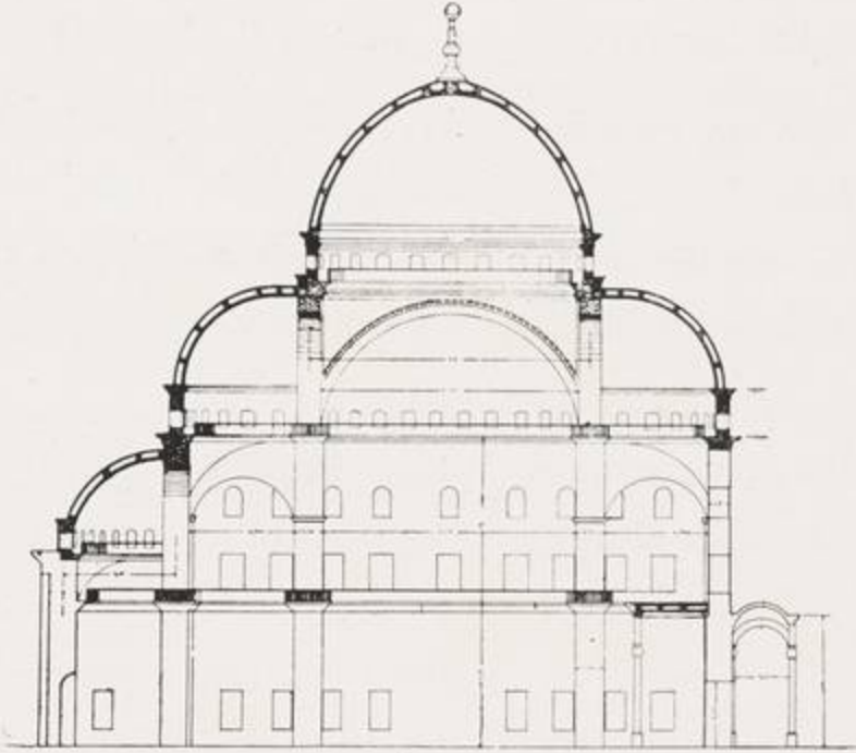
قطاع رأسي
