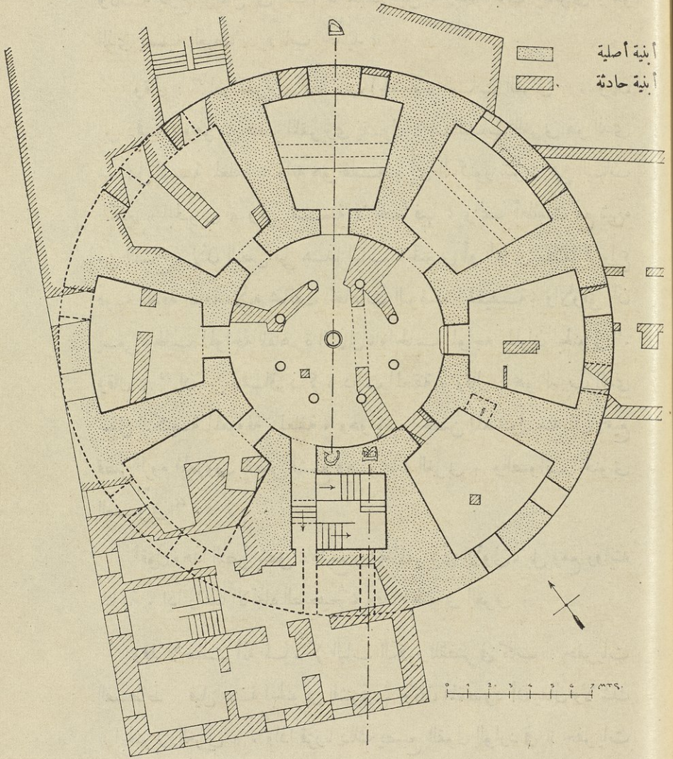
قطاع أفق لأحد البرجين الغربيين للمحصن الروماني (قصر الشمع) من محفوظات لجنة حفظ الآثار العربية
