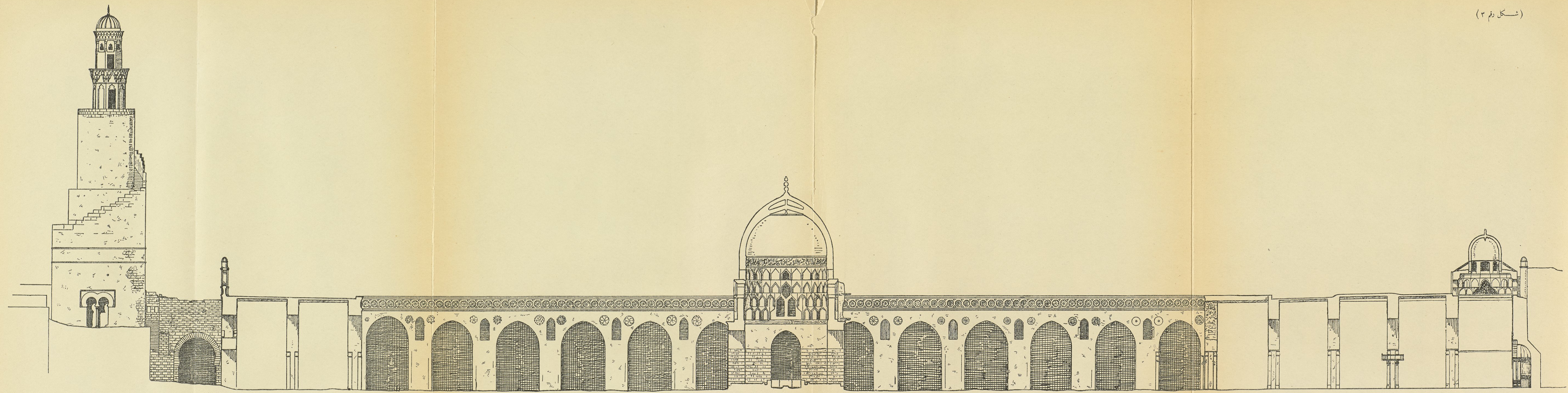
قطاع طولى للجامع بين المحراب والمنارة
