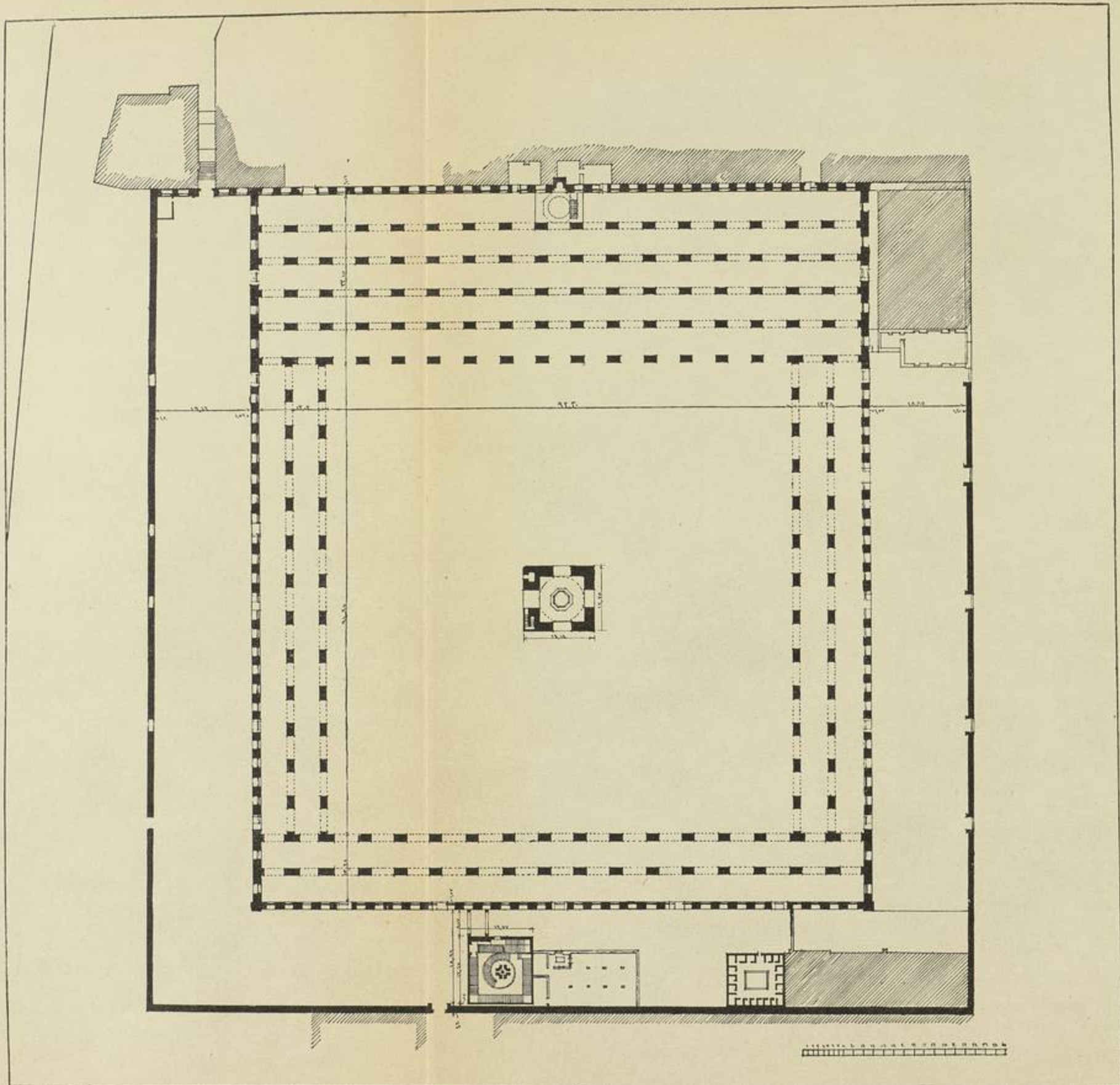
القطاع الأفقي للجامع
